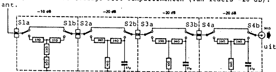
Fig. 1 -70 dB Stappenverzwakker
